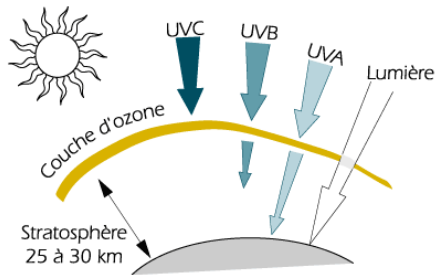
La couche d'ozone nous protège des rayons nocifs provenant du soleil / © Jean-Claude Puente
